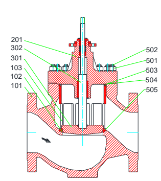
MV 5411-AR 2 , PV 6411-AR 2 with/ mit/ avec QCS NPS 10 - 12, CL 600
