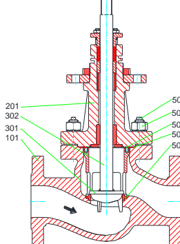
MV 5411-AR 1 , PV 6411-AR 1 with/ mit/ avec QCS NPS 1½ - 12, CL 600
