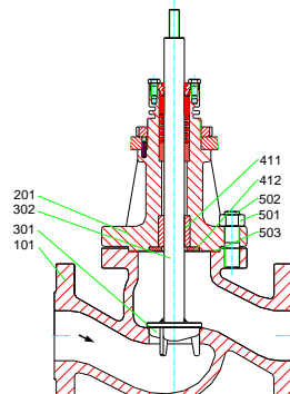
MV 5411-AR 1 , PV 6411-AR 1 NPS 1½ - 12, CL 600 - 900 3
