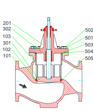
MV 5411-AR 2 , PV 6411-AR 2 with/ mit/ avec QCS NPS 10 - 12, CL 150 - 300
