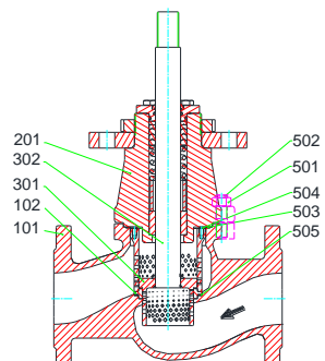
MV 5411-AR, PV 6411-AR with/ mit/ avec QCS 2-stage NPS 1½ - 6, CL 150 - 300
