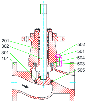
MV 5411-AR 1 , PV 6411-AR 1 with/ mit/ avec QCS NPS 1½ - 12, CL 150 - 300
